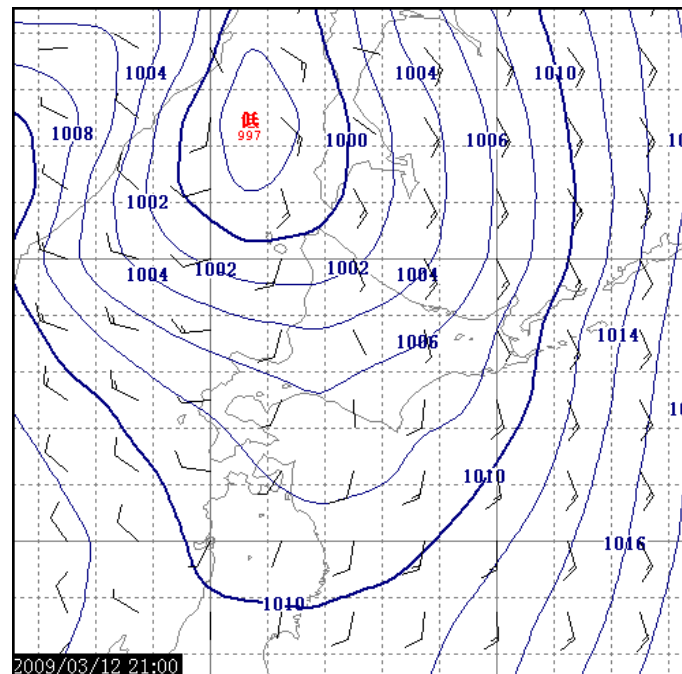
2009/03/12 21:00 T=192 等値線: 気圧(2hPa) 矢羽: 風向・風速(m/s)
