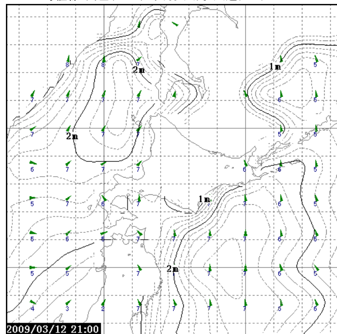
2009/03/12 21:00 T=192 等値線: 波高(0.2m) 矢じり: 波向 数値: 周期(s)
